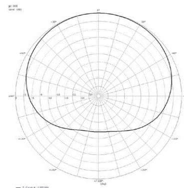
Polardiagramm @ 1 kHz
